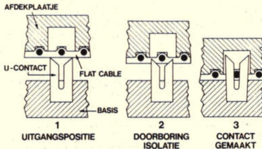
Fig. 1. Op deze manier wordt het zelfstrippende U-contact door de platte kabel geperst, waarna een uitstekende verbinding tussen kabelader tot stand komt. De afb. rechtsboven geeft een zgn. Delta-connector met behuizing voor deze techniek. Links een kabelconnector, die in een printconnector schuift en rechts het handpersje, waarmee alle typen connectoren aan de kabels worden bevestigd.
